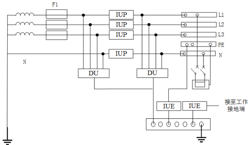
图6 TT系统隔离式装置的安装方式
