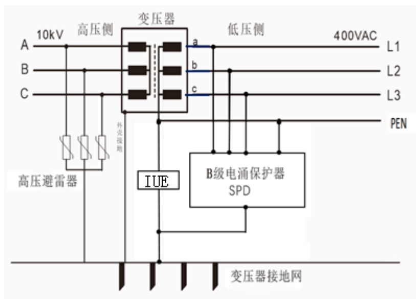
图8 变压器隔离式防护原理图
