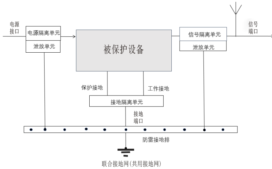
图5 隔离式防雷系统典型结构
