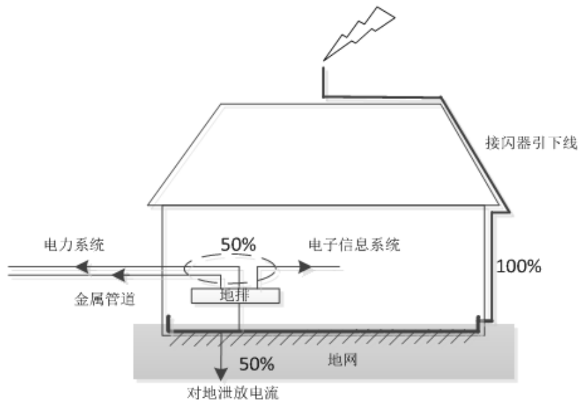
图3 采用统一接地方式的地电位反击分流比
