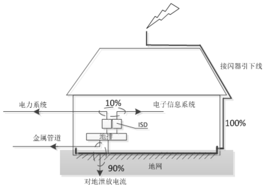
图4 采用分组接地方式的地电位反击分流比
