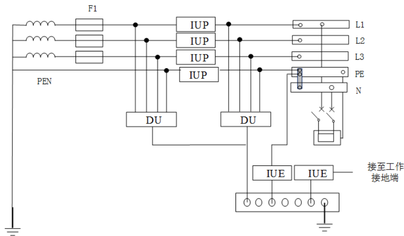
图7 TN系统隔离式装置的安装方式
